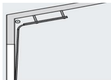
Направляющая ND со следованием по потолочному перекрытию
